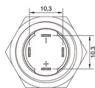
带灯按钮接线插片型(焊接脚)
